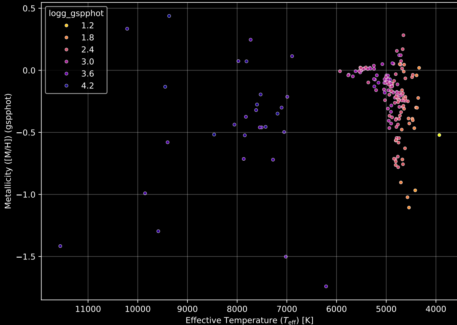
APOGEE DR17 Field: [180+19] Stellar Population Parameters (n= 182)
